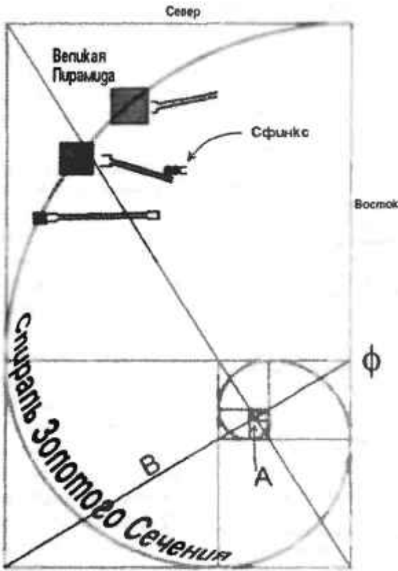
Рис. 11.1. Золотосеченная спираль. Символ \phi (фи) указывает точку, где правая вертикальная сторона делится по своей длине на два отрезка в пропорции \phi .
